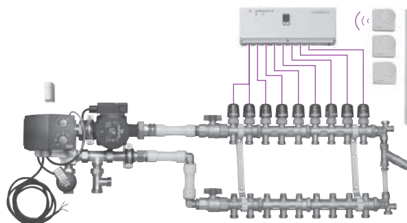
Uponor Push 45U Electronic med Uponor WGF 1" Fördelare och Uponor CoSy Radio rumsreglering.
