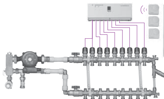
Uponor Push 45U med Uponor WGF 1" Fördelare och Uponor CoSy Radio rumsreglering.
